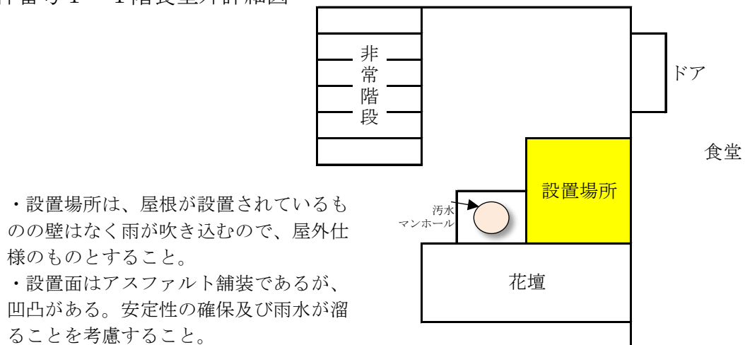
物件番号1 1階食堂外詳細図
